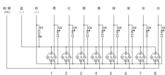
S010-M12-8 S011-M12-8
