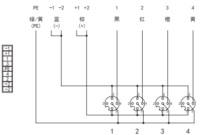
S012-M12-4C
