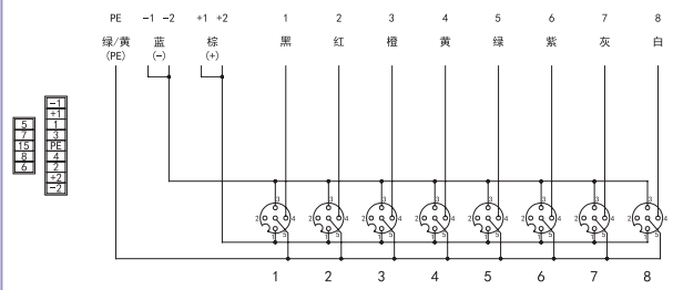
S012-M12-8C
