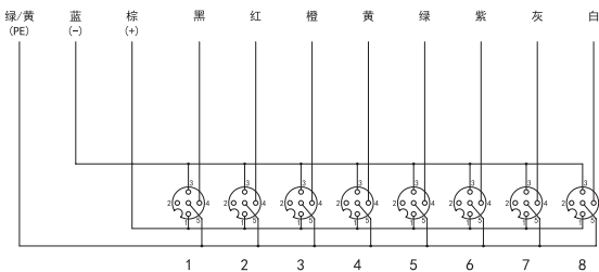
S010-M12-8C S011-M12-8C
